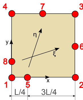
FIGURE 19.6: Position des nœuds de l'élément singulier de type Q8
