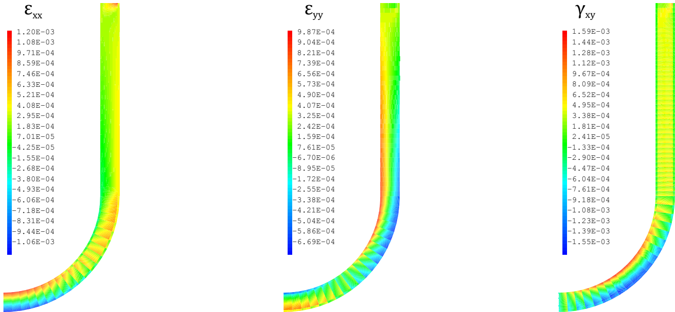
FIGURE 13.3: Déformations
