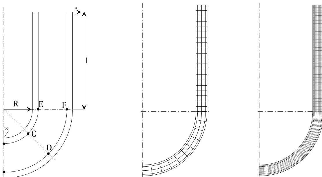
FIGURE 13.1: a) Géométrie de la poutre en U, b) le maillage utilisé pour le tester la méthode Reissner local, c) maillage permettant d'obtenir la « solution de référence » puisque'il n'y a pas de solution analytique
