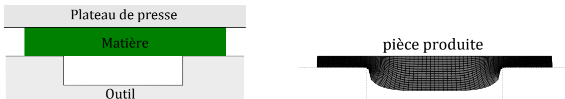
FIGURE 19.7: Thermocompression : a) problème, b) forme de la pièce après production
