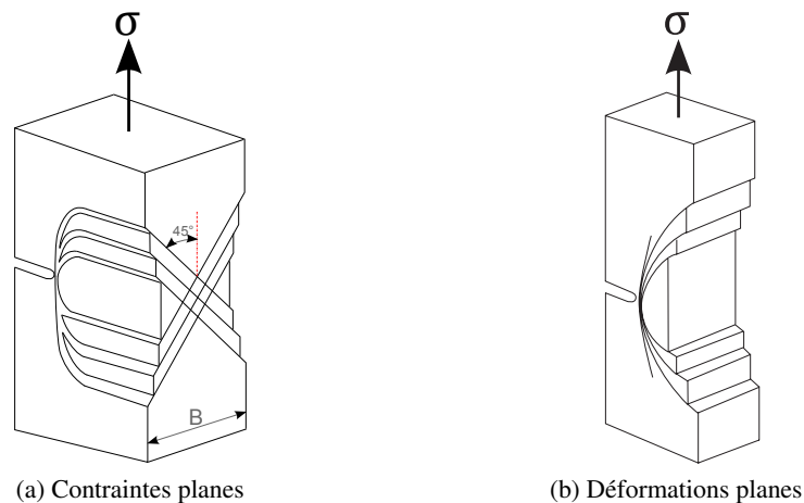
FIGURE 20.6: Zones de plastification d'une éprouvette entaillée en traction
