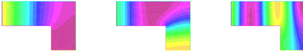
FIGURE 18.12: Avec condition de Neumann et pour des fréquences de 100, 500 et 1000 Hz
