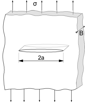
FIGURE 20.2: Concentration de contraintes autour d'une fissure : plaque mince
