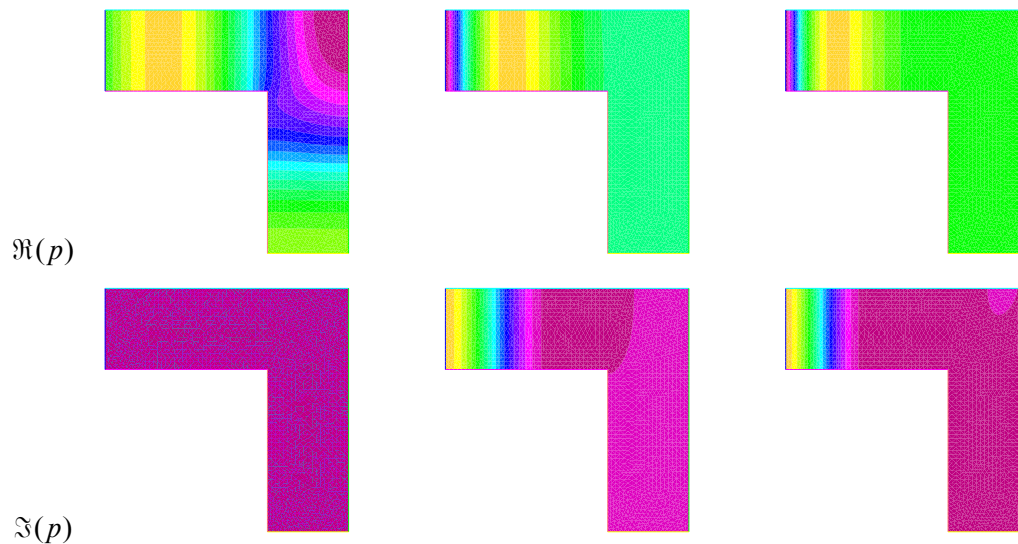
FIGURE 18.14: À 500 Hz avec un amortissement de 0, 1 et 2%
