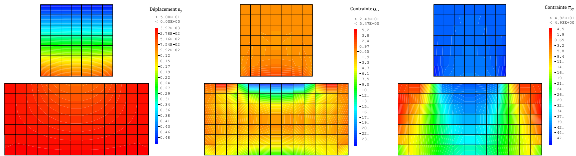
FIGURE 19.6: a) déplacement u_y b) \sigma_{xx} et c) \sigma_{yy}
