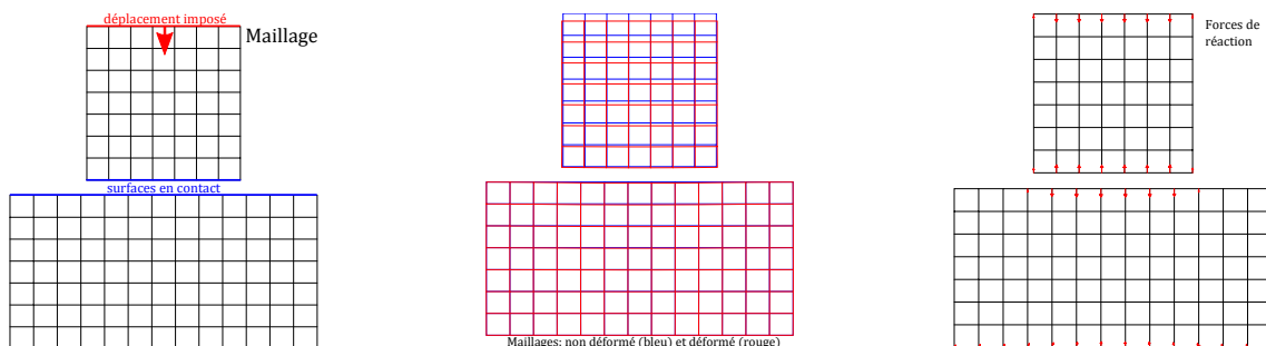
FIGURE 19.5: a) maillage, b) déformée c) forces de réaction
