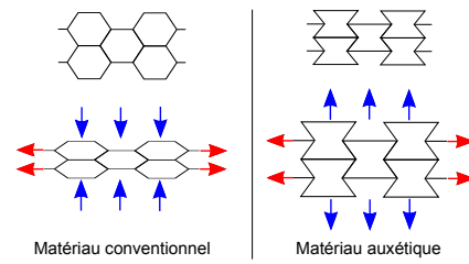
FIGURE 6.3: Matériau auxétique
