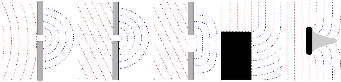
FIGURE 18.4: Phénomène de diffraction
