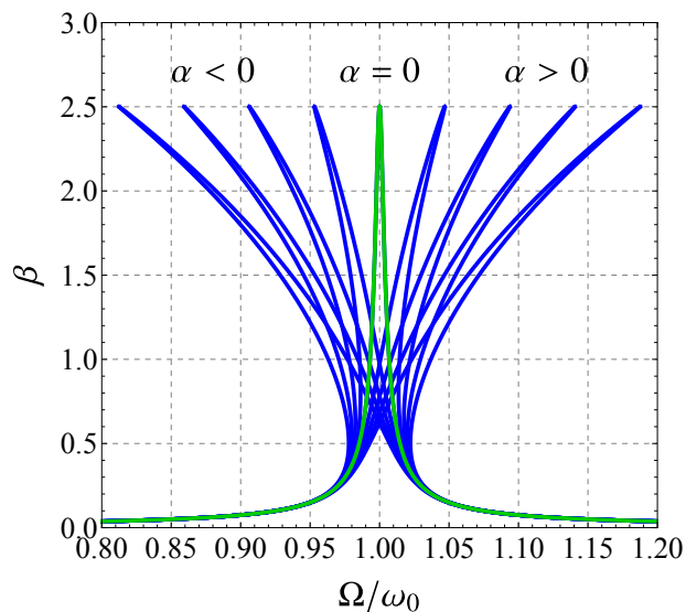
FIGURE 1.7. Réponse en fréquence d'un oscillateur de Duffing pour différente valeur de \alpha .
