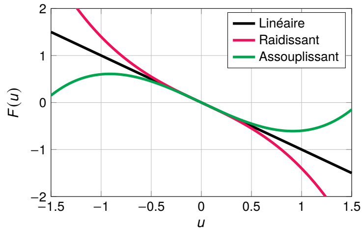
FIGURE 1.5. Force de rappel d'un ressort linéaire (ligne noire), d'un ressort dont la non-linéarité est raidissante (ligne rouge) et d'un ressort dont la non-linéarité est amortissante (ligne verte).
