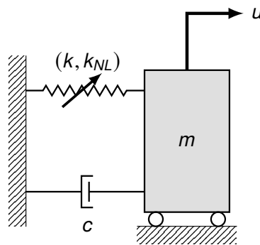
FIGURE 1.6. Système masse-ressort avec amortisseur visqueux et force de rappel non linéaire.
