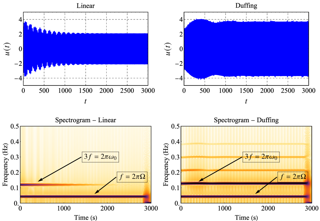
FIGURE 1.8. Illustration du phénomène de résonance super-harmonique. À gauche le cas linéaire et à droite le cas non linéaire. À chaque fois il y a en haut la série temporelle de u(t) , issue de l'intégration numérique de (1.11), et en bas le spectrogramme correspondant.
