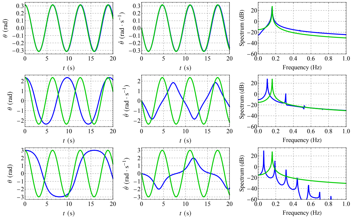
FIGURE 1.3. Simulations numériques de (1.1) (bleu) et de l'équation linéarisée correspondante \ddot{\theta} + \frac{g}{\ell}\theta = 0 (vert). Première colonne : série temporelle de \theta ; deuxième colonne : série temporelle de \dot{\theta} et troisième colonne : périodogramme.
