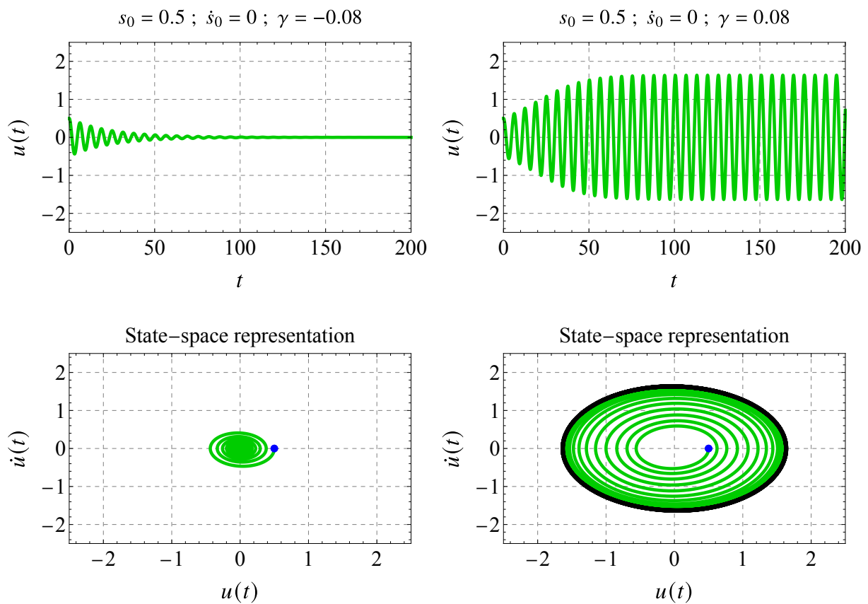
FIGURE 1.11. Intégration numérique de (1.16) avec \gamma = -0.08 à gauche, \gamma = 0.08 à droite et \alpha = 0.04 . En haut : Série temporelle. En bas : représentation dans l'espace des phases. Les trajectoires sont représentées en vert et, dans l'espace des phases, le cycle limite est représenté par une ligne noire et la condition initiales par un point bleu.
