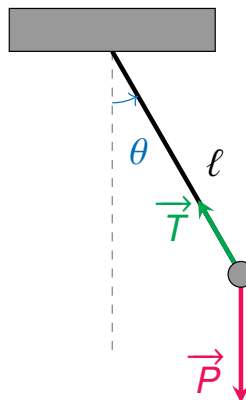
FIGURE 1.2. Pendule pesant.
