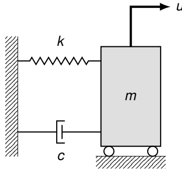
FIGURE A.3. Système masse-ressort avec amortisseur visqueux.
