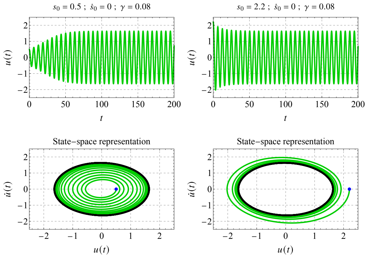
FIGURE 1.12. Intégration numérique de (1.16) avec \gamma = 0.08 et \alpha = 0.04 . En haut : Série temporelle. En bas : représentation dans l'espace des phases. À gauche conditions initiales sont à l'intérieur du CLO. À droite conditions initiales sont à l'extérieur du CLO. Les trajectoires sont représentées en vert et, dans l'espace des phases, le cycle limite est représenté par une ligne noire et la condition initiales par un point bleu.
