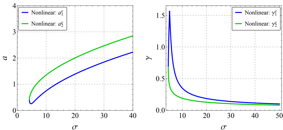
FIGURE 3.8. Points fixes de (3.44) : amplitudes a^e (à gauche) et phases \gamma^e (à droite). Les paramètres suivants sont utilisés : \mu = 0.3 , \alpha = 5 et K = 5 .
