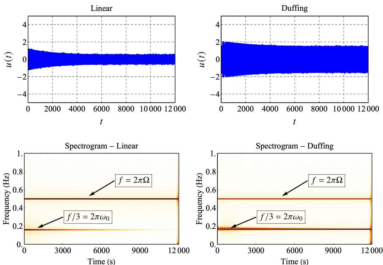
FIGURE 1.9. Illustration du phénomène de résonance sous-harmonique. À gauche le cas linéaire et à droite le cas non linéaire. À chaque fois il y a en haut la série temporelle de u(t) , issue de l'intégration numérique de (1.11), et en bas le spectrogramme correspondant.
