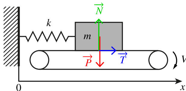
FIGURE 1.10. Modèle phénoménologique simple permettant de reproduire des vibrations induites par le frottement.
