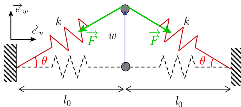
FIGURE 1.4. Déplacement transversal w de deux ressorts linéaires de raideur k .
