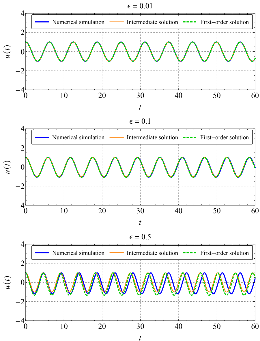
FIGURE 2.5. La solution intermédiaire (2.141) et celle à l'ordre 1 (2.140) sont comparées à l'intégration numérique directe de (2.62) pour s_0 = 1 et (de haut en bas) \epsilon = 0.01, 0.1 et 0.5 . De plus \alpha_2 = 1 et \alpha_3 = 2 .
