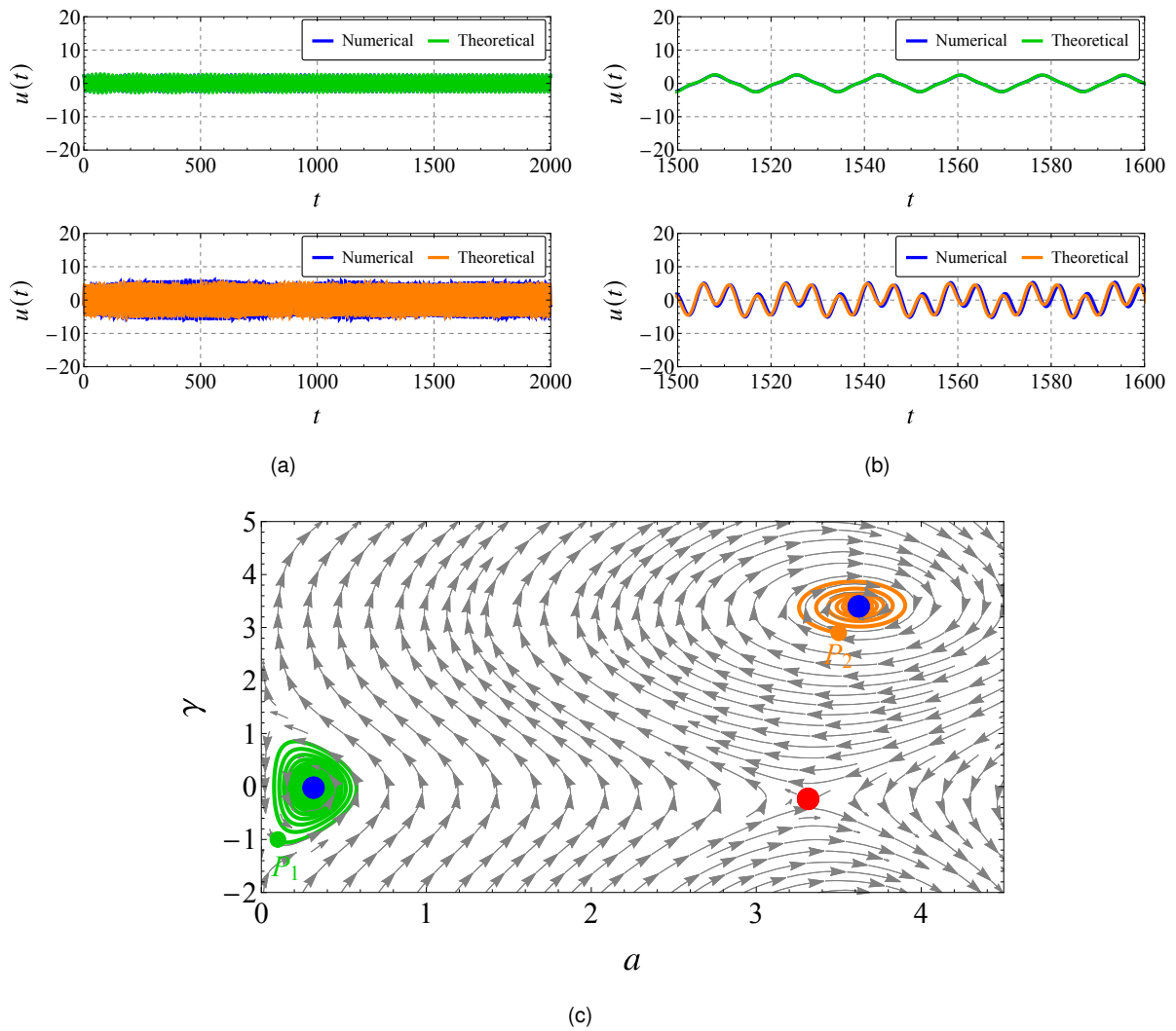
FIGURE 3.6. Intégration numérique des systèmes (3.4) et (3.36) pour \sigma = 25 et pour deux conditions initiales P_1 = (0.1, -1) et P_2 = (3.5, 2.9) . La figure montre (a) u en fonction du temps et (b) la trajectoire dans le plans (a, \gamma) comparé aux lignes de champ de (3.36). Les points bleus et rouge représentent respectivement les points fixes stables et instable. Même paramètres que dans la Fig. 3.5 avec \epsilon = 0.003 . (b) Zoom de la Fig. 3.6(a) entre t = 1500 et t = 1600 .
