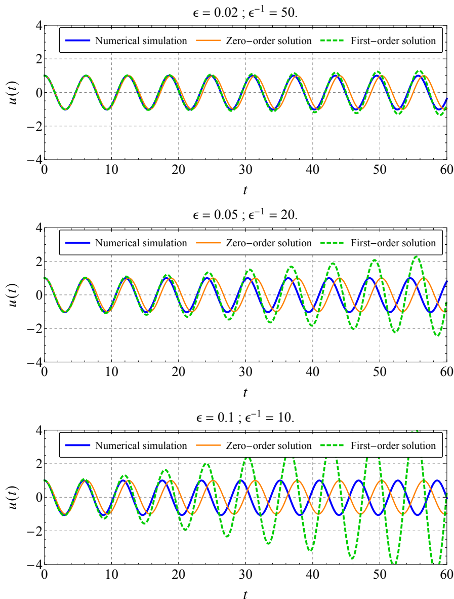
FIGURE 2.3. Résultat de la méthode des perturbations « naïve ». Les solutions aux ordres 0 (i.e. Éq. (2.70), solution du système linéaire associé) et 1 (i.e. Éq. (2.89)) sont comparés à l'intégration numérique directe de (2.62) pour s_0 = 1 et (de haut en bas) \epsilon = 0.01, 0.05 et 0.1 . De plus \alpha_2 = 1 et \alpha_3 = 2 .
