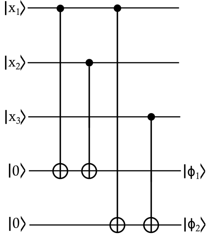
Fig. V.9. Error correcting code.
