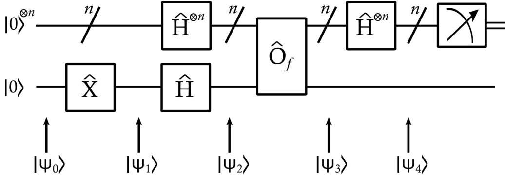
Fig. III.17. Implementation Deutsch-Joza algorithm.
