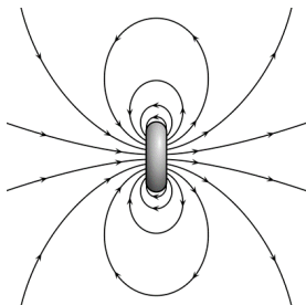
Dipôle Magnétique
